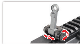
照門旋鈕(左/右調整)
